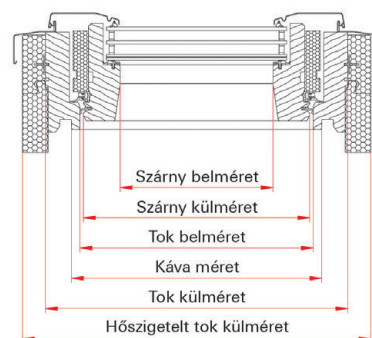
B-B metszet
