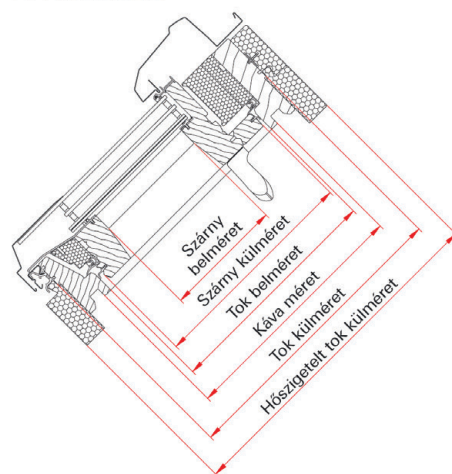
B-B metszet
