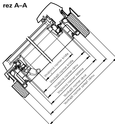
rez A-A
