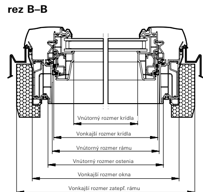
rez B-B
