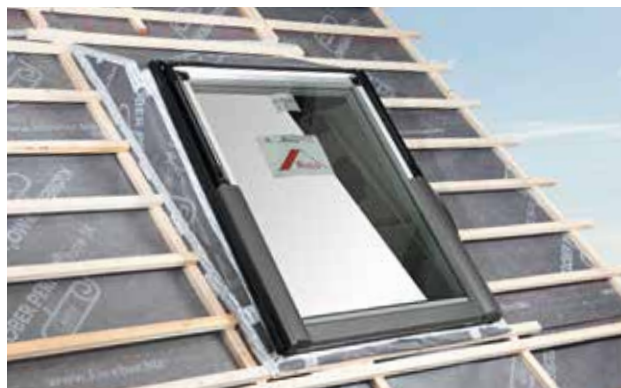
Možnosť použitia pri sklone strechy od 15 stupňov.
