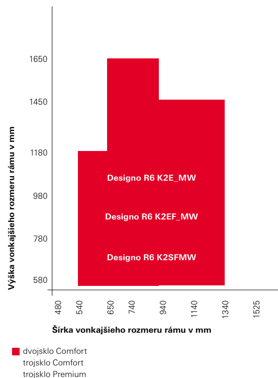
Tabuľka rozmerov - elektrické okno na mieru MW
