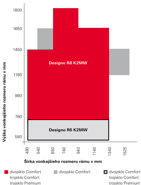
Tabuľka rozmerov - manuálne okno na mieru MW
