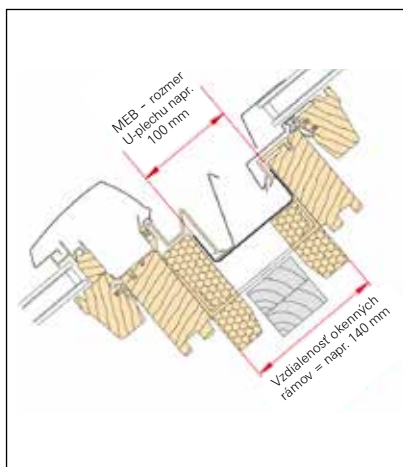
Rez oknom R4/R7
