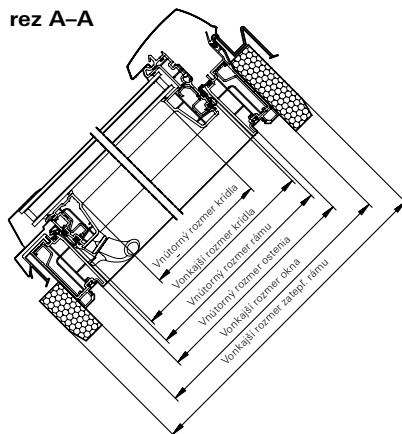
rez A-A
