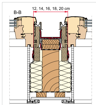
Štandardná kombinácia bez pomocnej krokvy EKS
