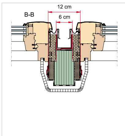
Kombinácia pomocnej krokvy EKS s napojením na systémové ostenie Roto ZIN
