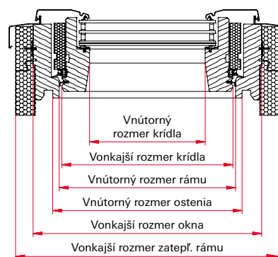
Rez B-B
