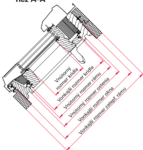
Rez A-A
