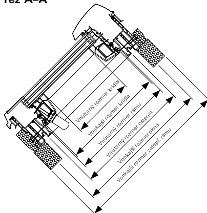
rez A-A
