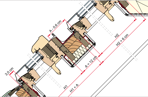
Accoppiata verticale RotoQ: distanza esterno telaio 120 mm Simulazione di montaggio standard. Verificare valori riportati in tabella.
