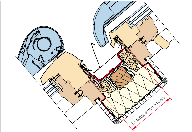
Accoppiata verticale R6/R8: distanza esterno telaio 140 mm Simulazione di montaggio standard. Verificare valori riportati in tabella.
