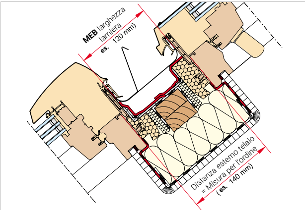
Accoppiata verticale R6/R8: larghezza MEB con distanza esterno telaio 140 mm Simulazione di montaggio standard. Verificare valori riportati in tabella.
