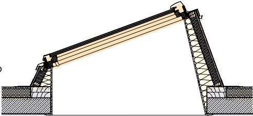
Particolare raccordo per tetti piani: + 20°
