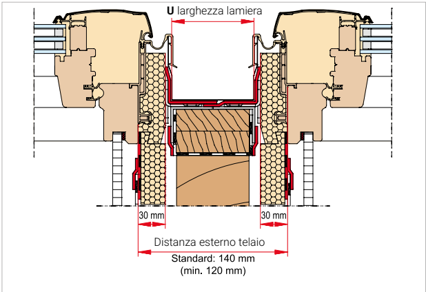
Accoppiata orizzontale R6/R8: larghezza UBL con distanza esterno telaio 140 mm. Simulazione di montaggio standard. Verificare valori riportati in tabella.
