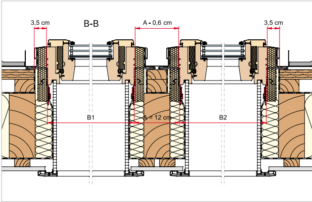
Accoppiata orizzontale RotoQ: distanza esterno telaio 120 mm Simulazione di montaggio standard. Verificare valori riportati in tabella.
