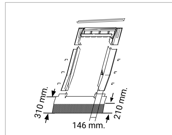
Quote profili scossalina per finestre Designo
