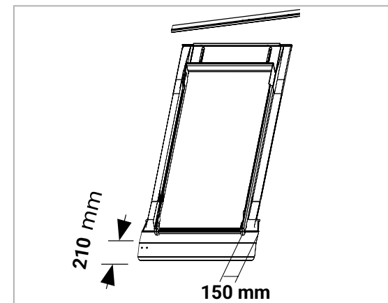
Quote profili scossalina per finestre RotoQ
