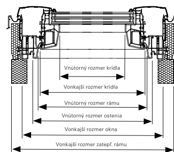
rez B-B
