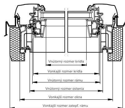
rez B-B
